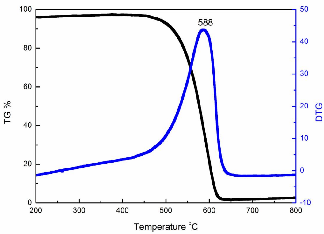
TGA
