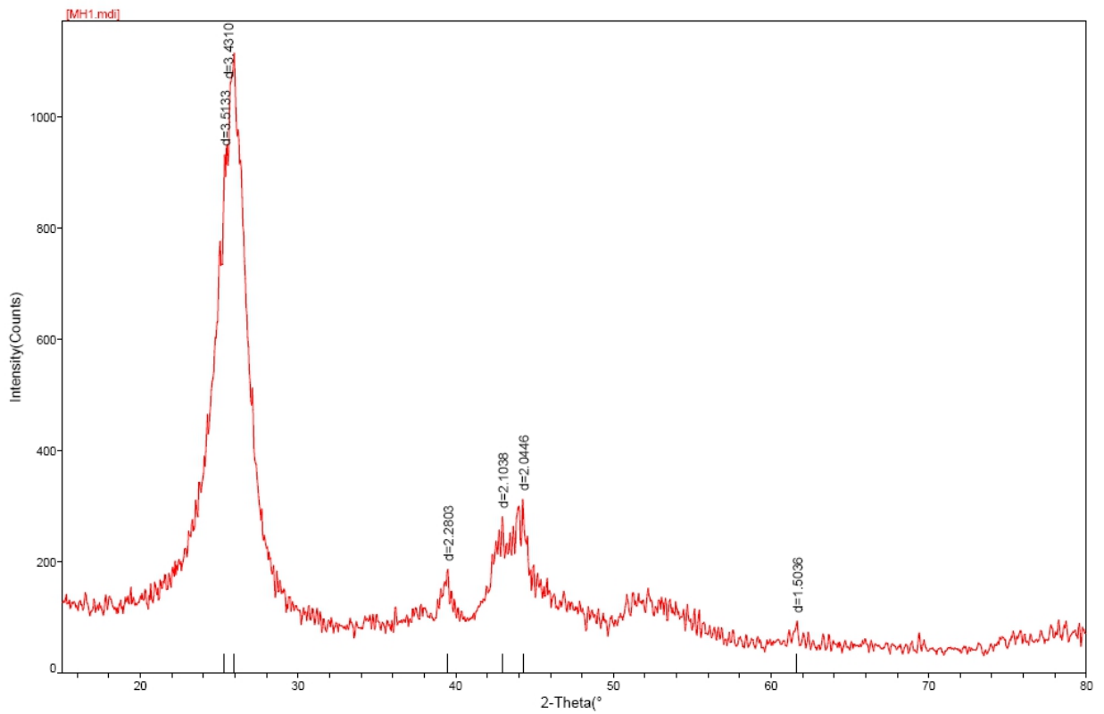
XRD
